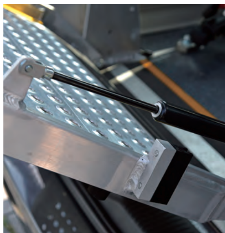
Euro Ramp 活動式斜坡板 （* 可另外選用可旋轉式活動坡道）（本圖示車型為 All-New Caravelle）
