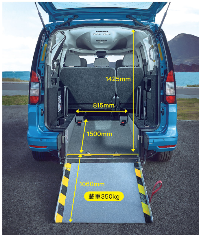
* 放下便捷省力的斜坡板
