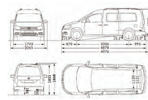
車身尺寸圖
