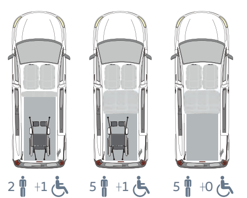
座位配置圖
